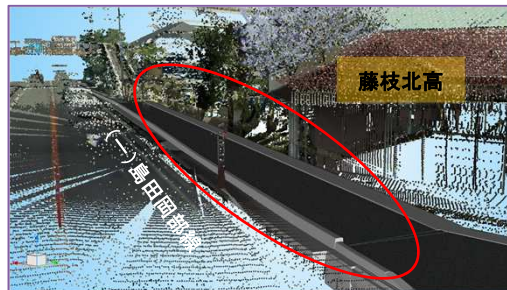
施工後（3次元モデル）
