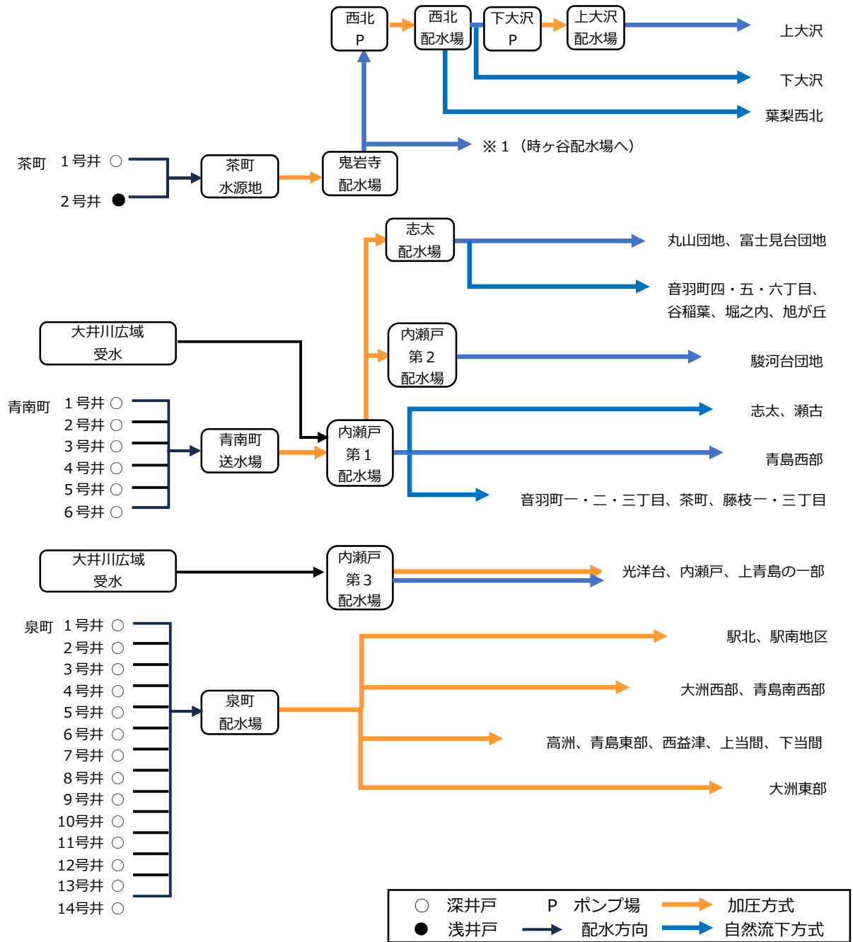
図 3.2 施設の系統図その1
