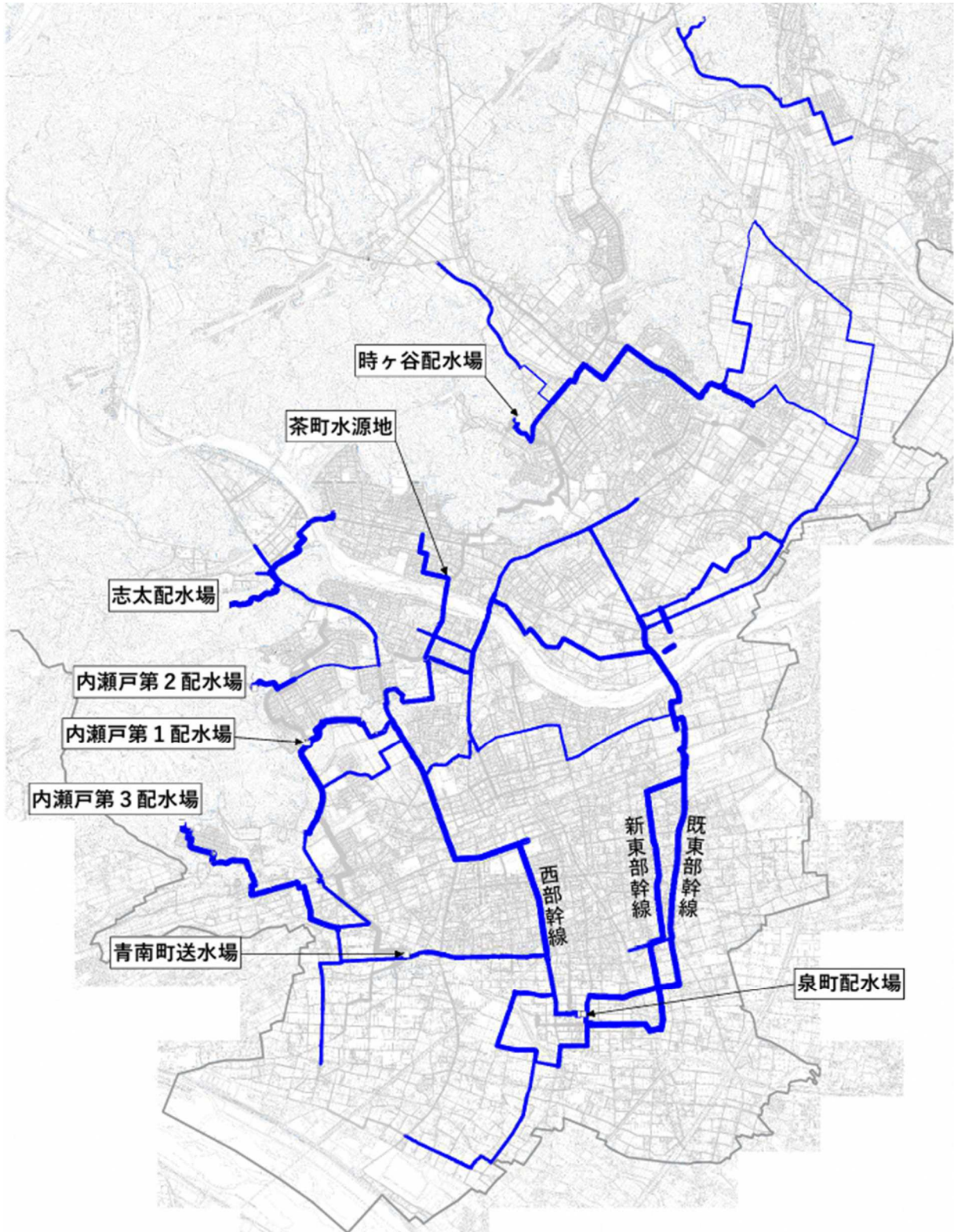
図 3.5 配水本管の配置状況(令和6年度)
