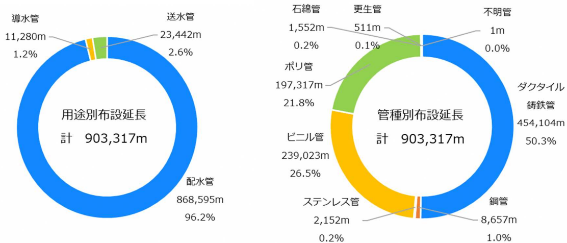
図 3.4 管路構成
