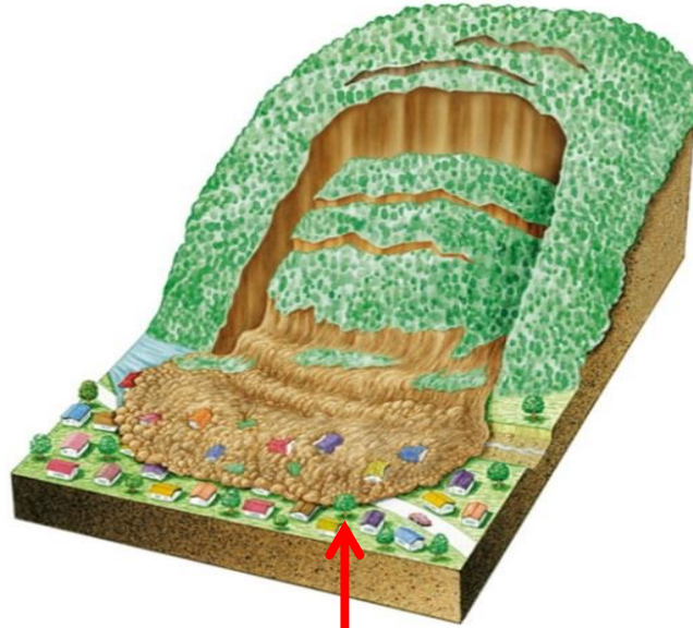
じ 地すべり
