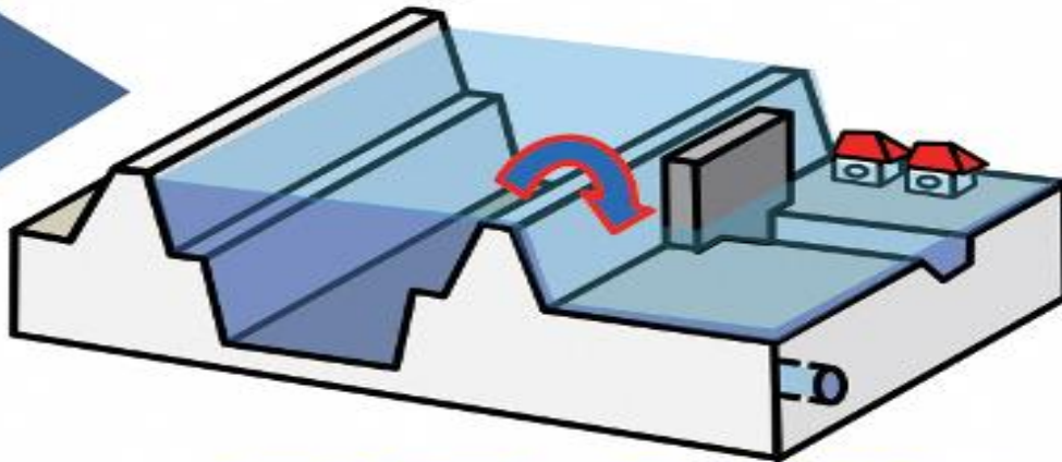
水位が堤防の高さを越える
