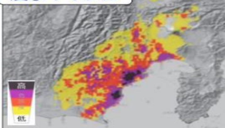
浸水キキクル
