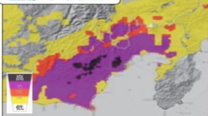
土砂キキクル
