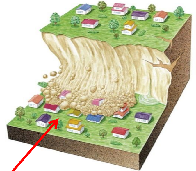
くず がけ崩れ ※急傾斜地崩壊
