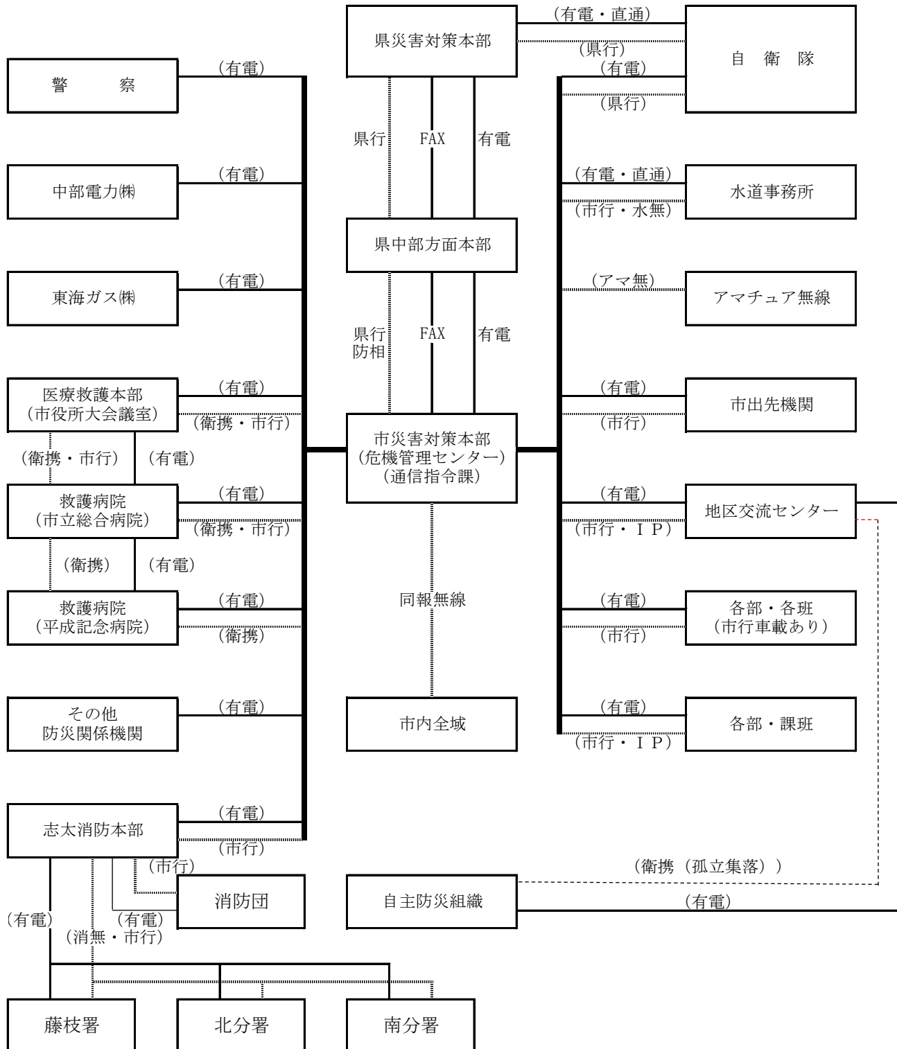
資料1-3 防災情報通信系統図
