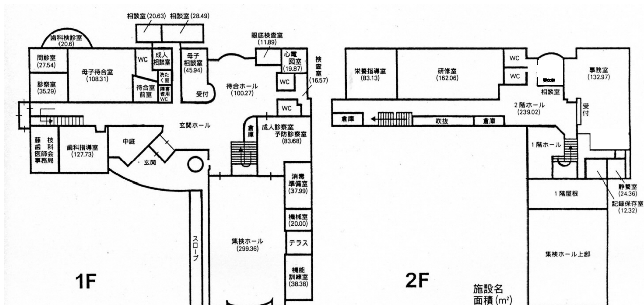
配置図及び平面図
